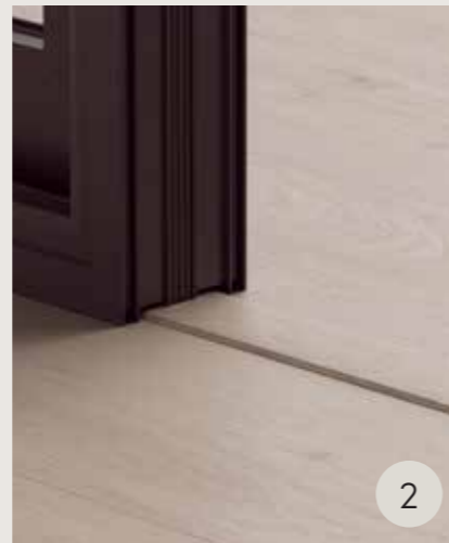
PROFILO DI DILATAZIONE 2000 x 38 x 8 mm Per coprire il giunto di dilatazione tra due pavimenti della stessa altezza.
