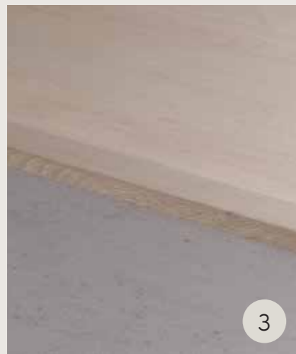
PROFILO DI TRANSIZIONE 2000 x 45 x 8 mm Per coprire il giunto di dilatazione tra un pavimento più alto e uno più basso.
