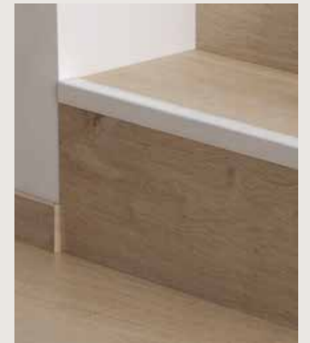
PROFILO PER SCALE, ARGENTO 2500 x 30 x 25 mm Per pavimenti di spessore 7 - 15 mm. Alluminio. PGSTPSILVME250
